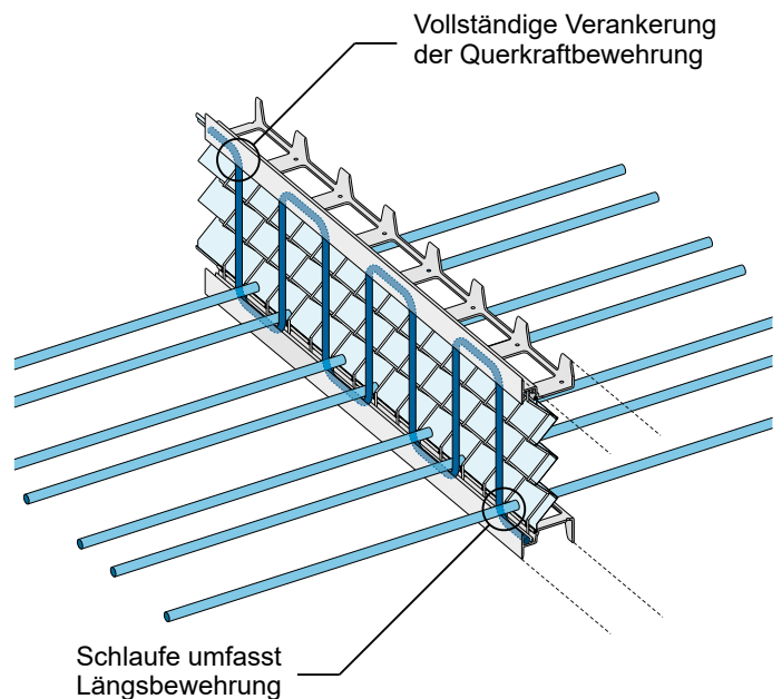
Bild 3: Abschalungselement: Vorzüge der Schlaufenbewehrung.
