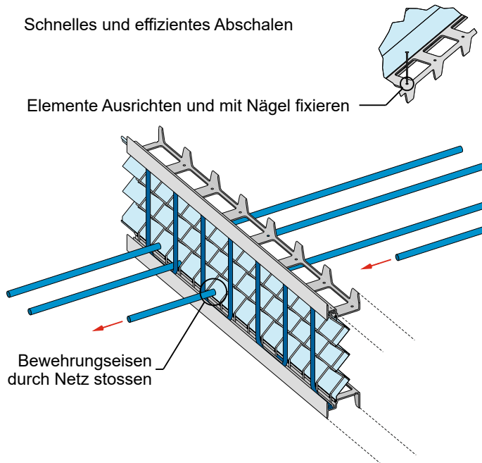
Bild 2: Abschalungselement: Verlegen.
