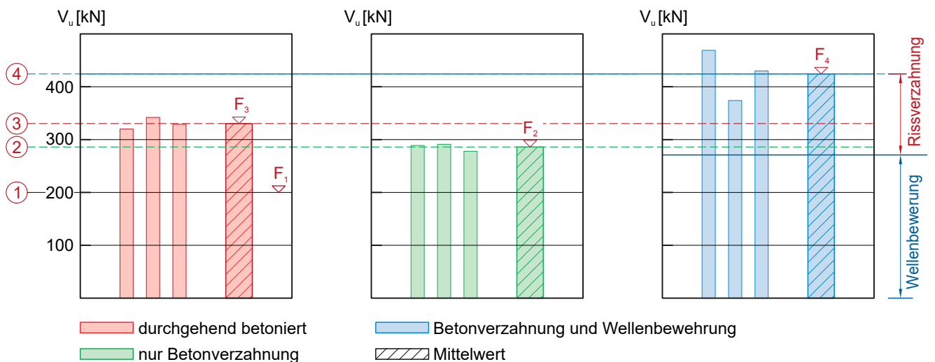
Bild 5: Darstellung der experimentellen Versuchsergebnisse: durchgehend betoniert (rot), Abschalungselement nur Betonverzahnung (grün), Abschalungselement mit Betonverzahnung und Schlaufenbewehrung (blau).
