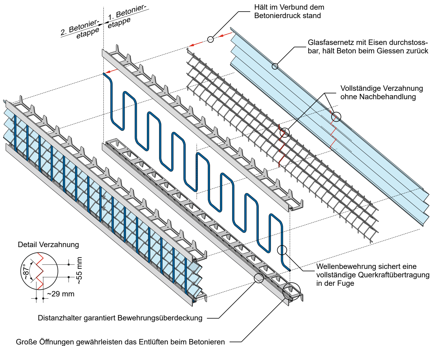
Bild 1: Abschalungselement: in axonometrischer Darstellung; Darstellung der Bauteile in Explosionsdarstellung.
